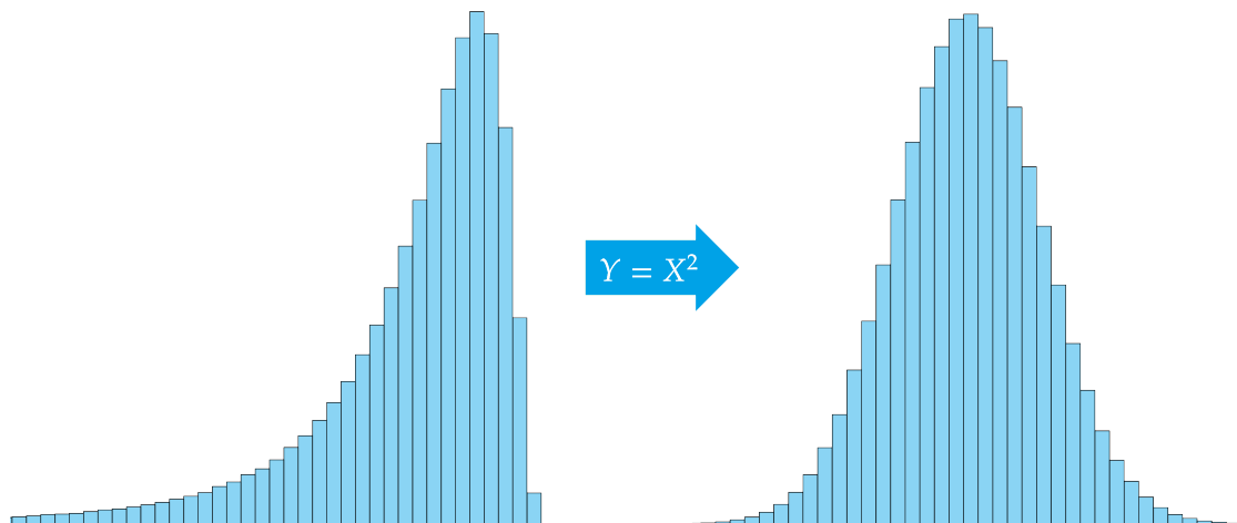
Figura 2.27: Transformación cuadrática.
