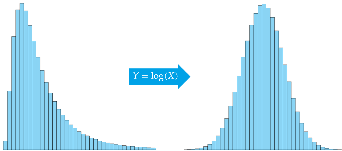
Figura 2.28: Transformación logarítmica.
