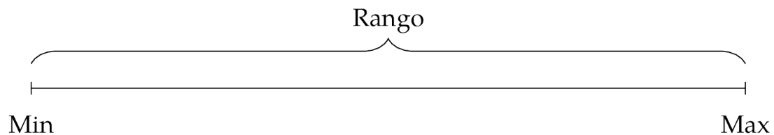
Figura 2.12: Rango muestral.
